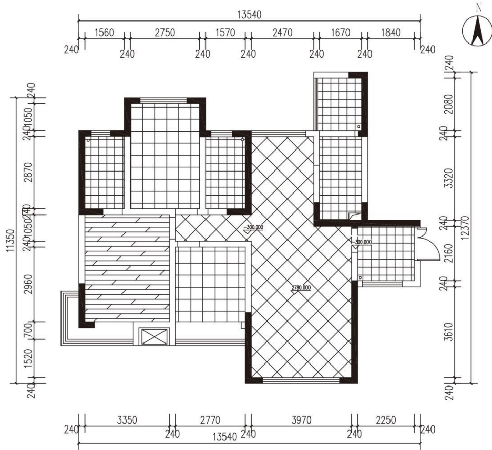
地面铺装图1:100
