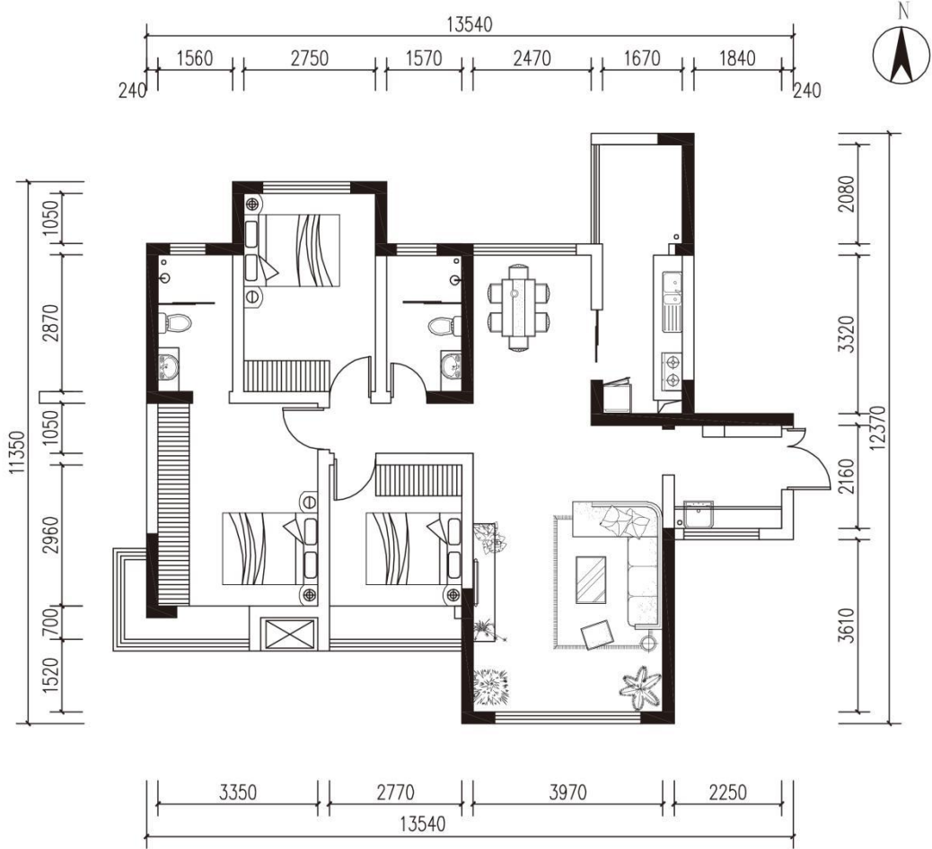
平面布置图 1:100
