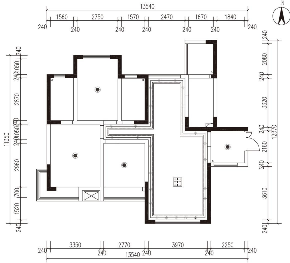
吊顶设计图 1:100
