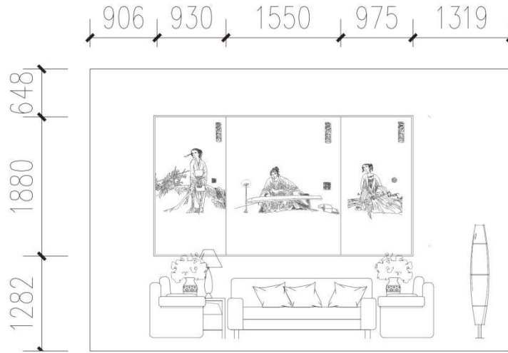
沙发背景墙立面图
