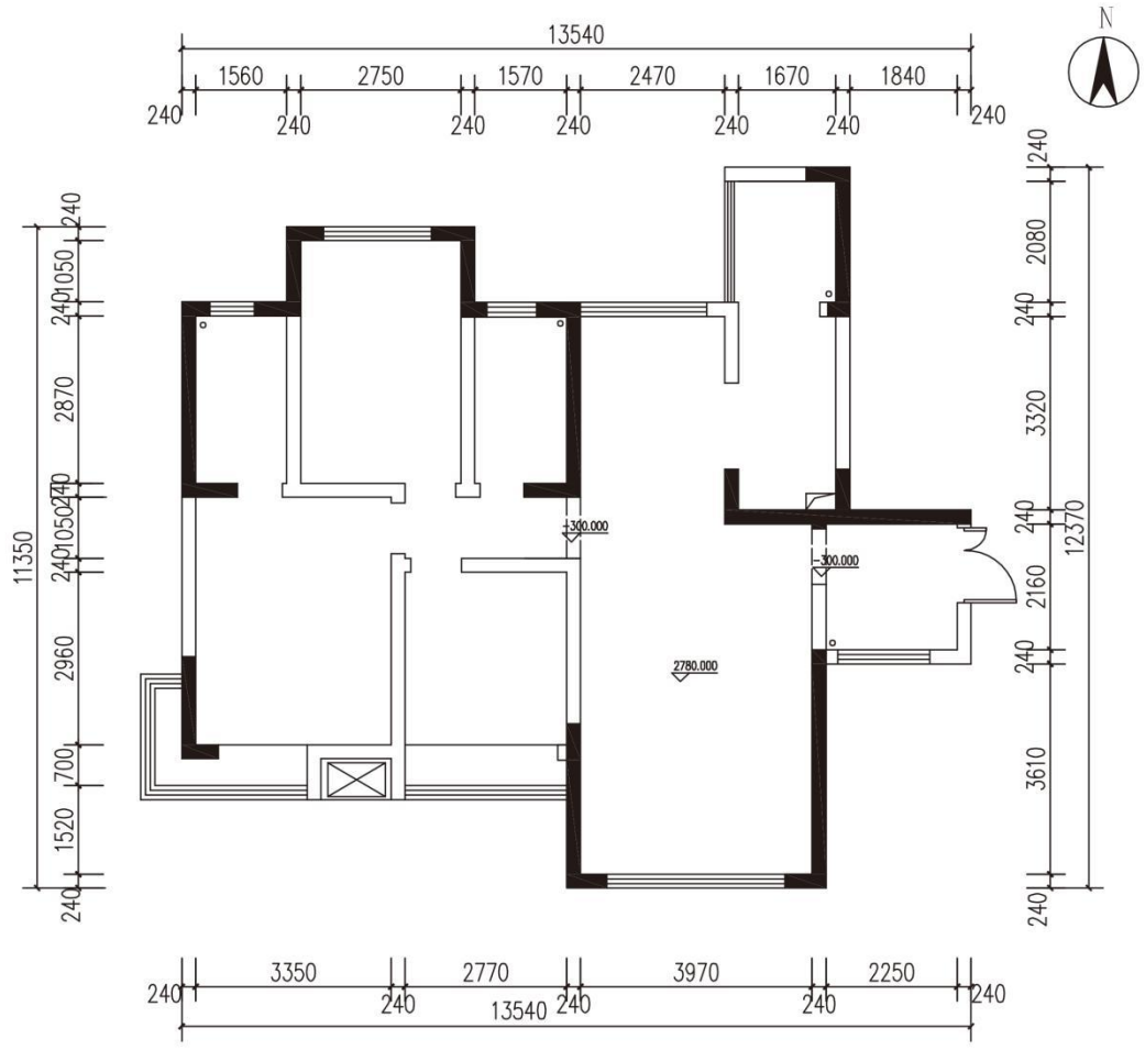
原始平面图 1:100
