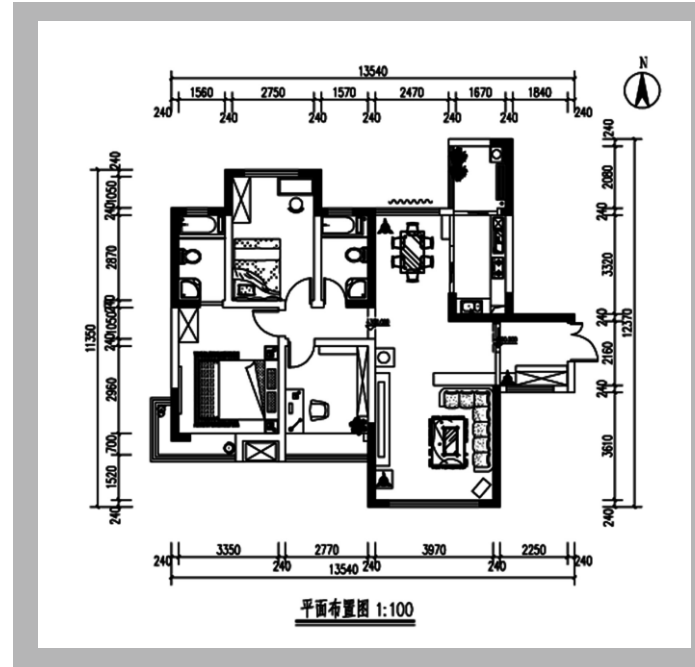
平面展示图 ▼
