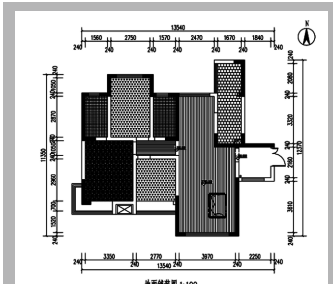
地面铺装图 ▼
