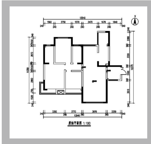
原始平面图 ▼
