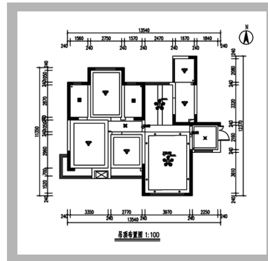
吊顶布置图 ▼
