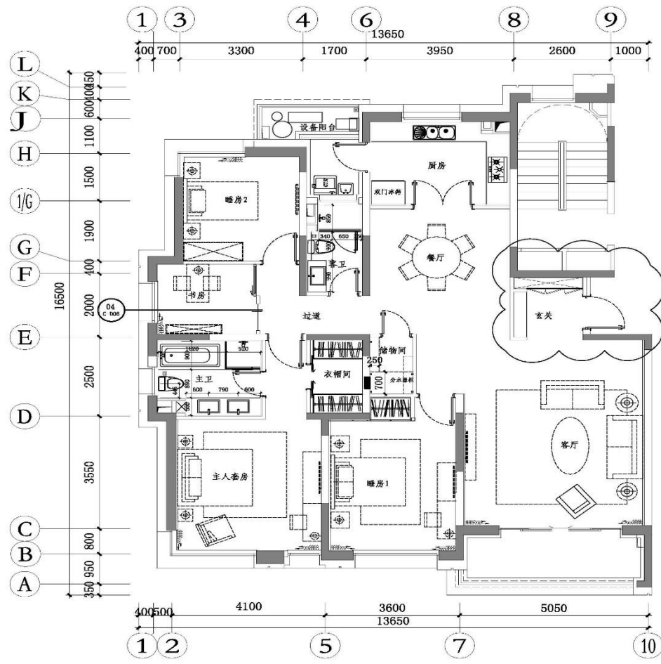
C 户型平面布置图
